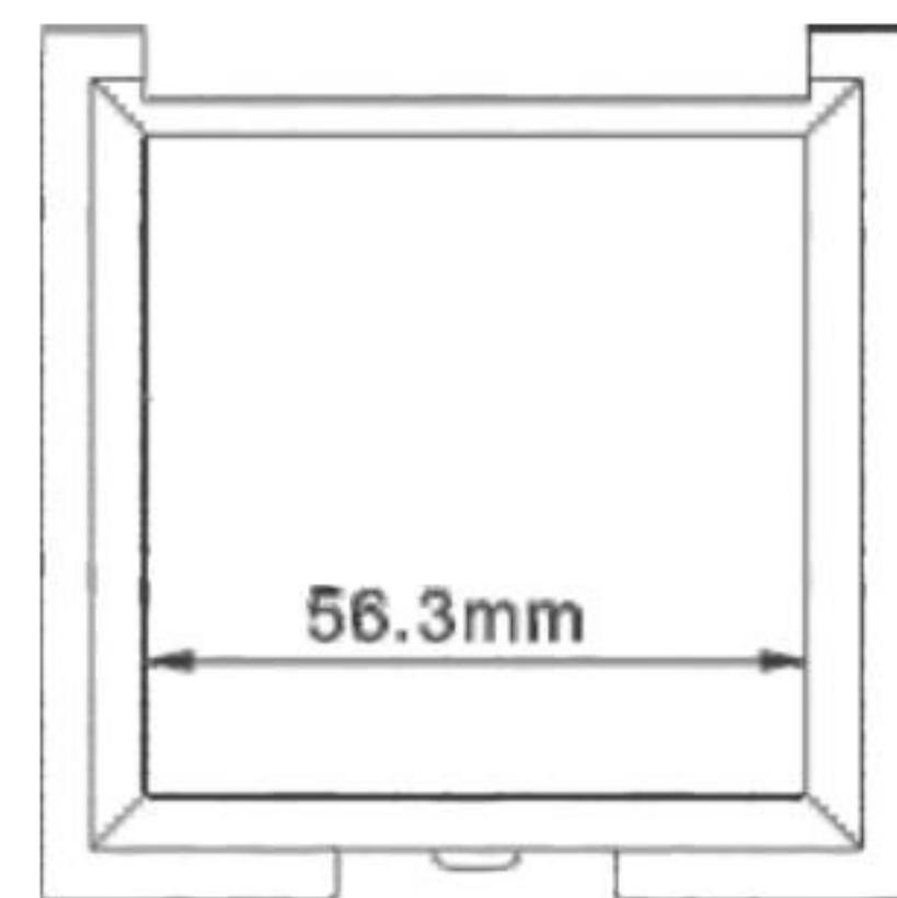
HG7141A SIZE:L70.5*W70.5*H16.8MM
