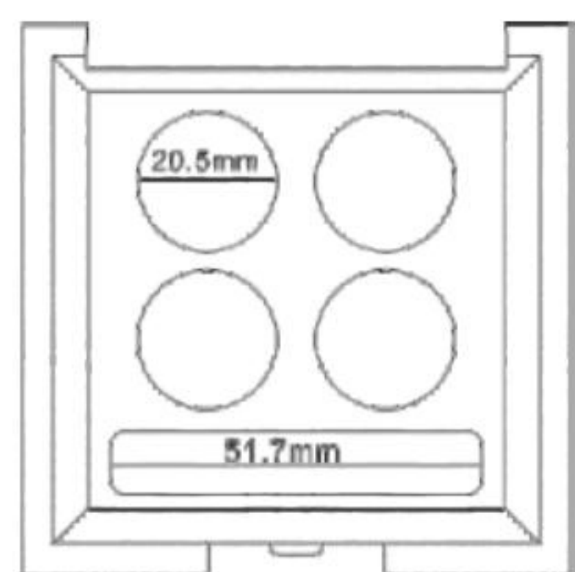
HG7141B SIZE:L70.5*W70.5*H16.8MM
